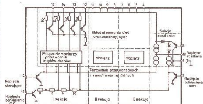
Rys. 5. Schemat ideowy układu scalonego A277D
