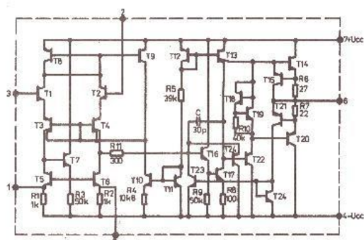
Rys. 4. Schemat ideowy układu scalonego ULY7741N
