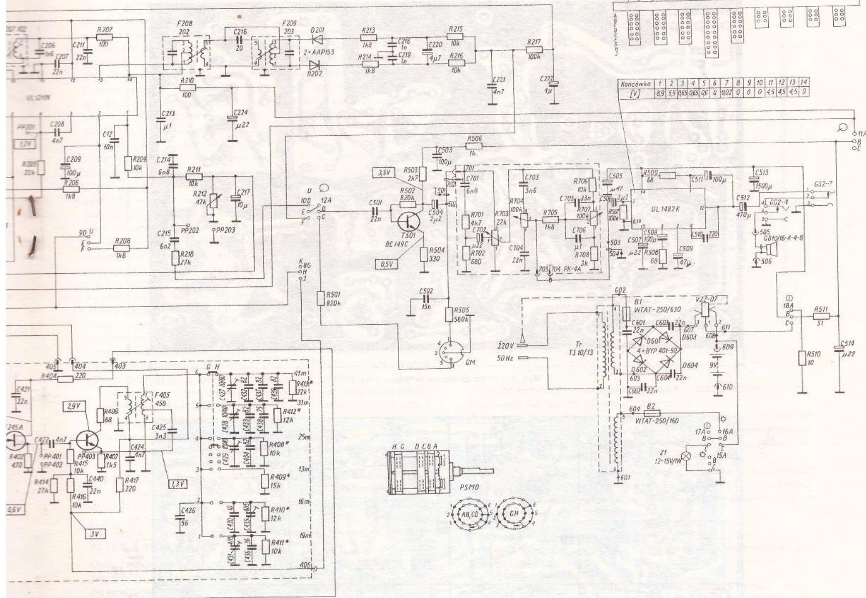
Schemat odbiornika radiofonicznego SABINA R610
